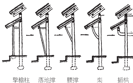
图二 檐部结构
