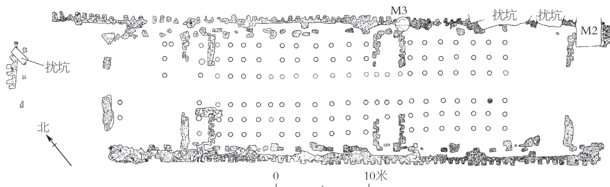
图一 青关山 F1 建筑遗址平面图 (采自《四川文物》2020年第5期)
