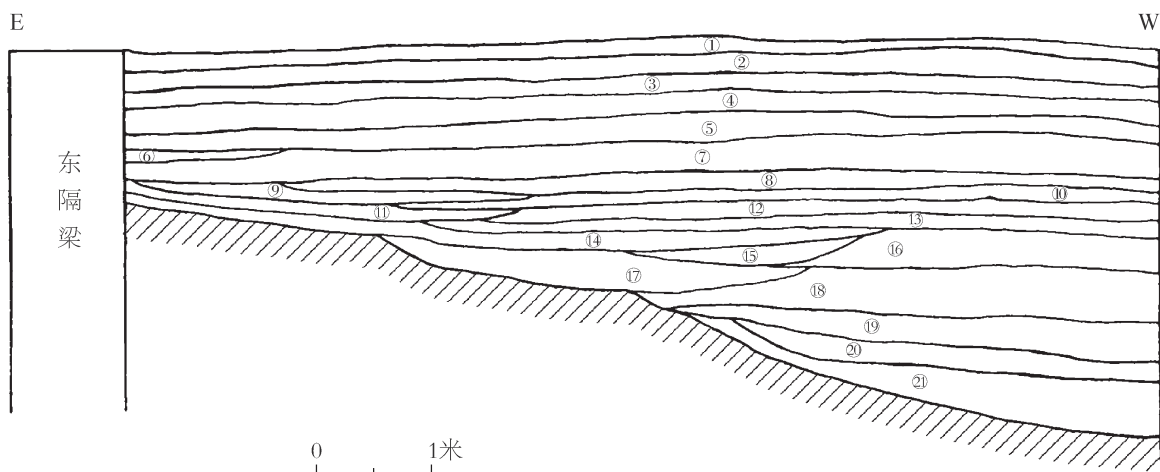
图三 TS03W13 南壁剖面图
