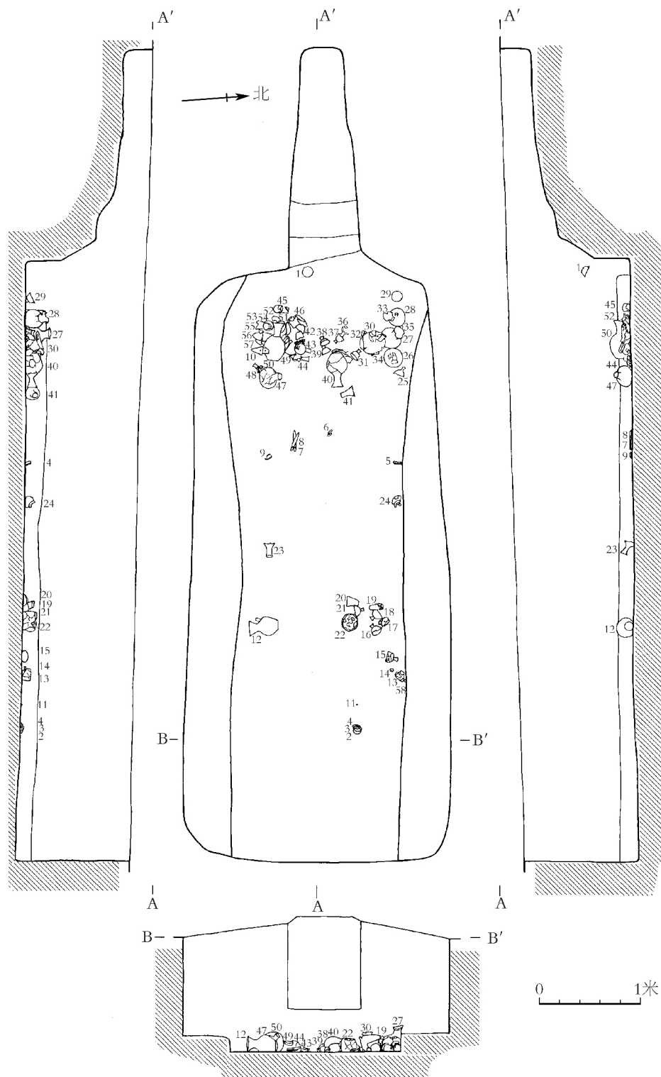
图一七 M118 平、剖面图
