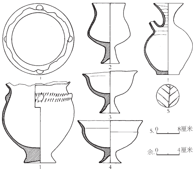
图一〇 M119 出土陶器
