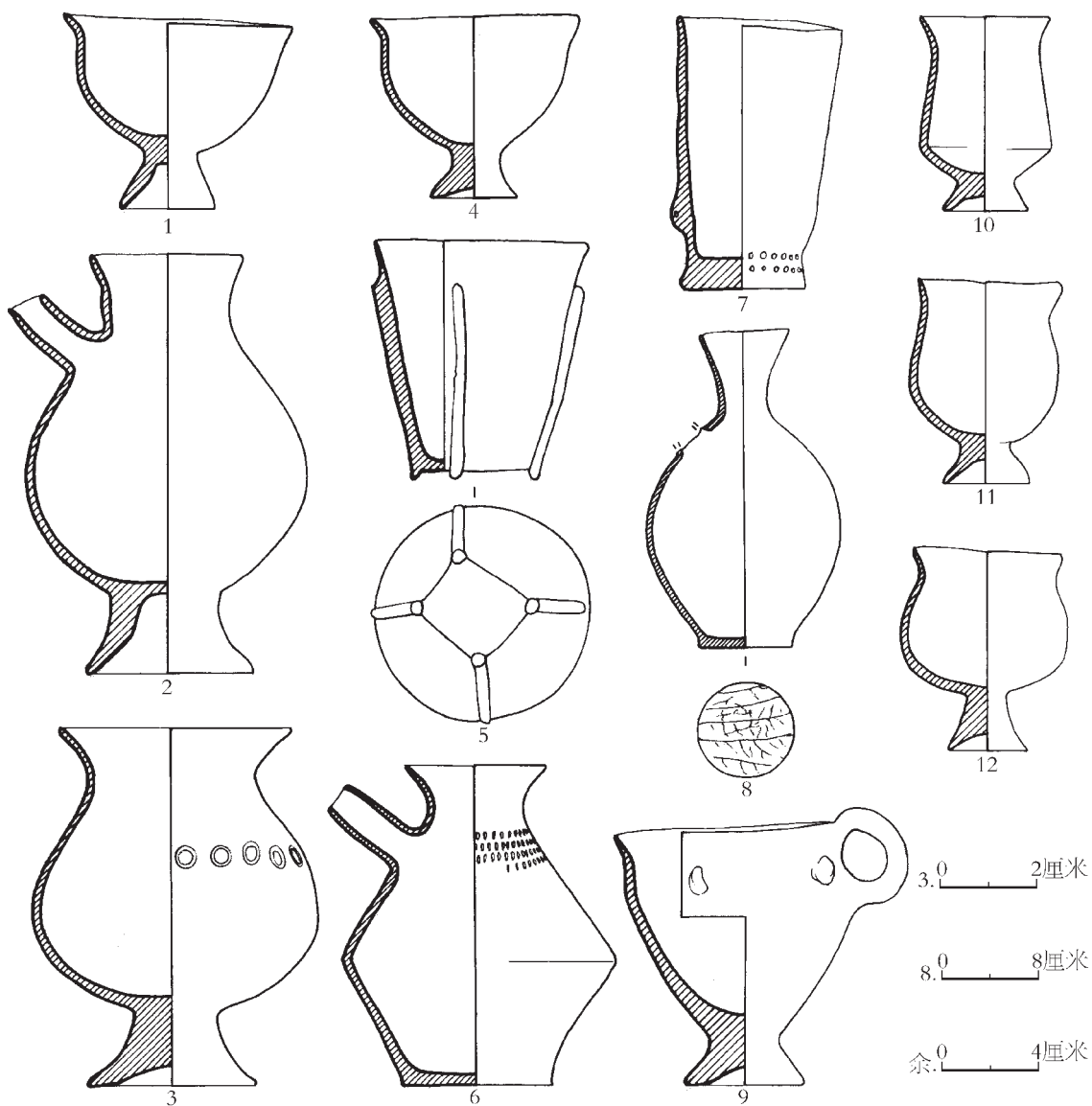
图一五 M116 出土陶器
