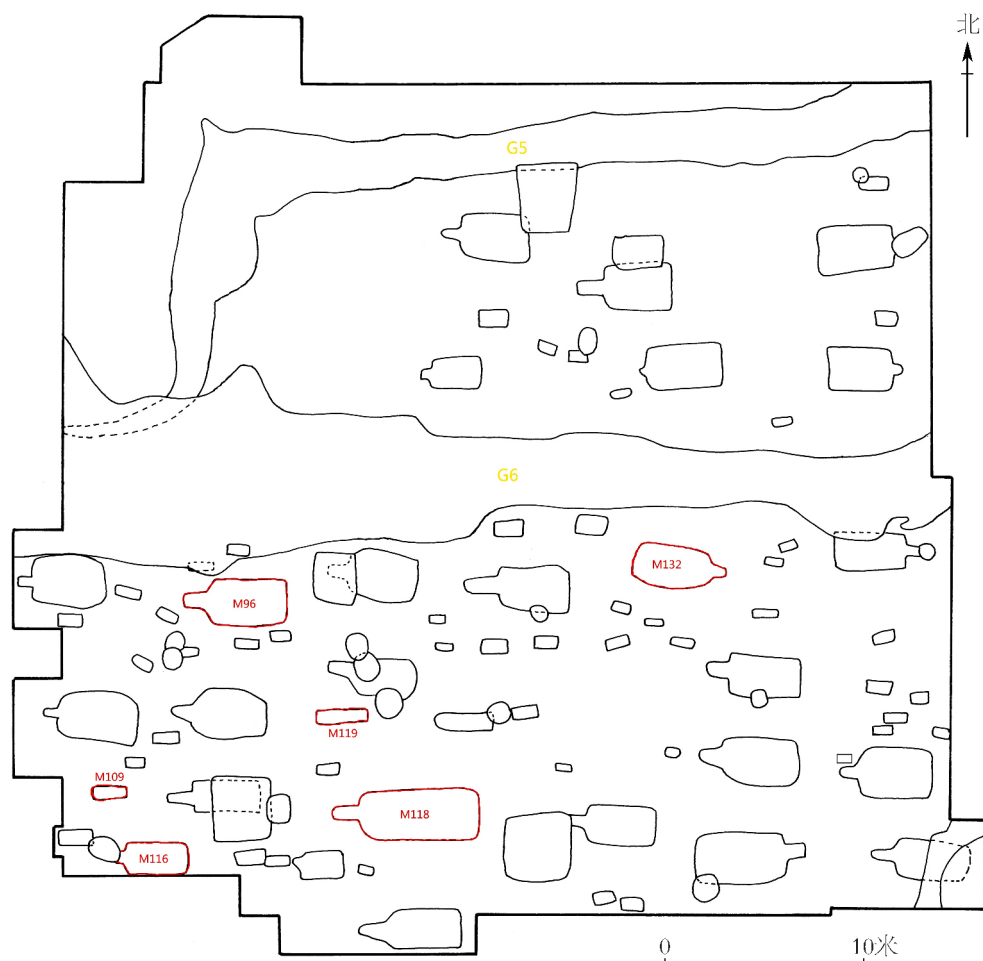
图三 槽子田墓地墓葬分布图
