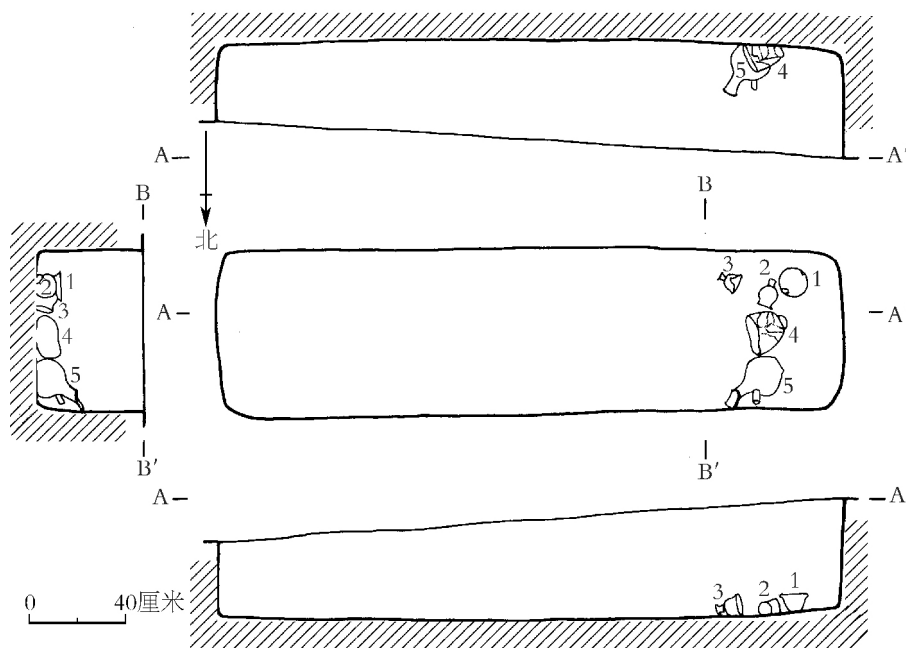
图九 M119 平、剖面图
