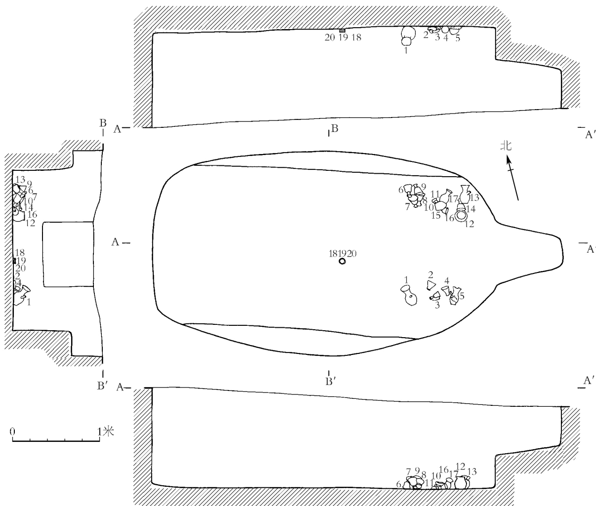
图二一 M132 平、剖面图
