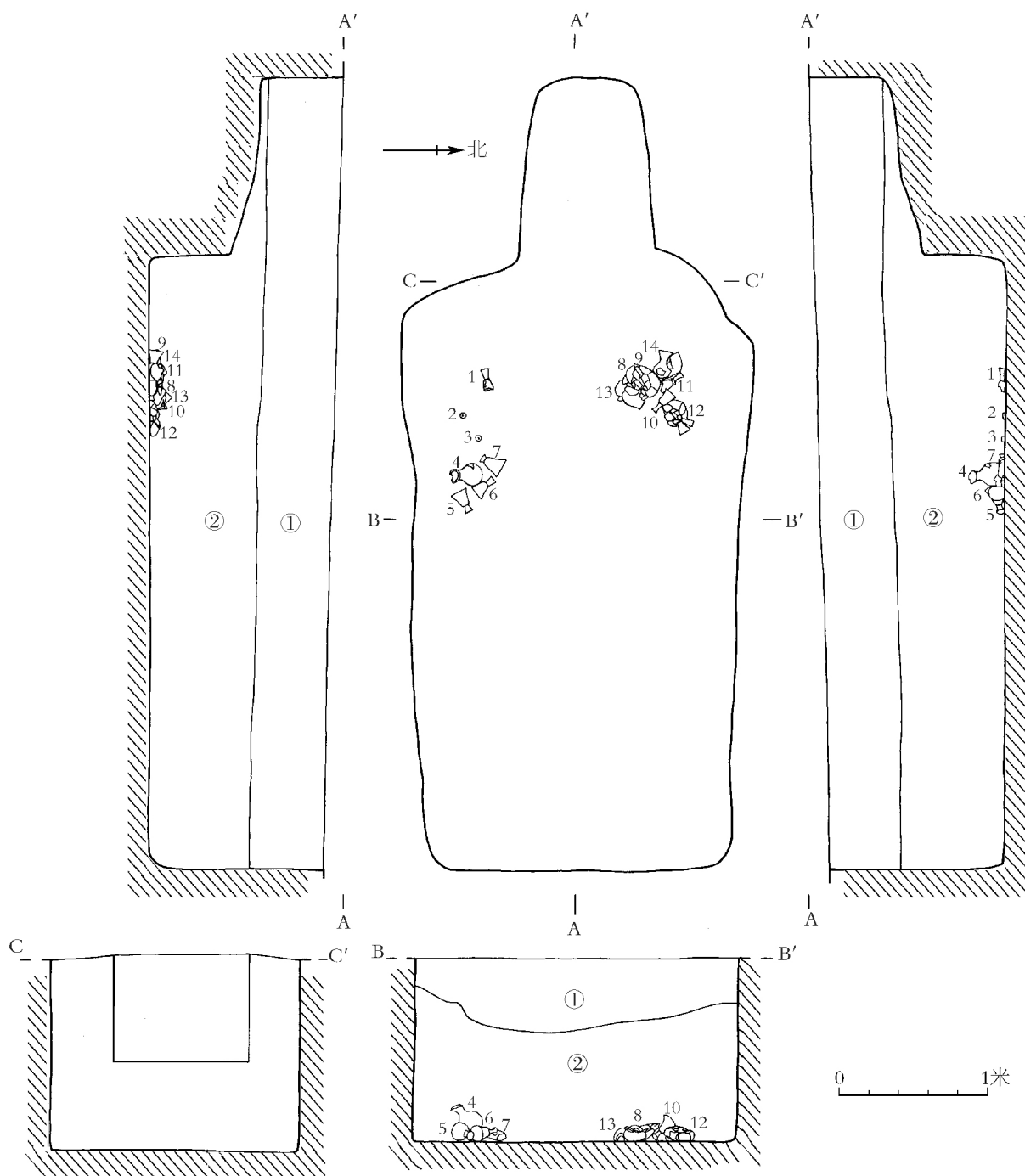
图一二 M96 平、剖面图
