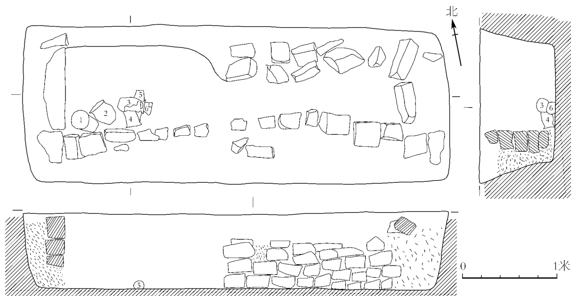
图二〇 M370 平、剖面图
