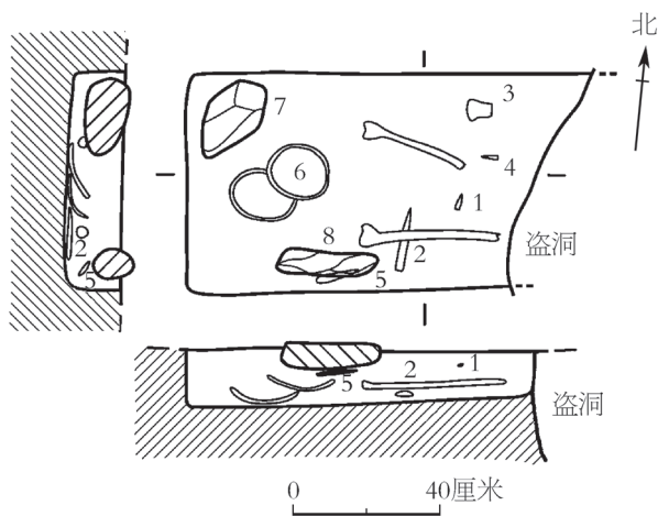
图三 M1 平面、剖视图
