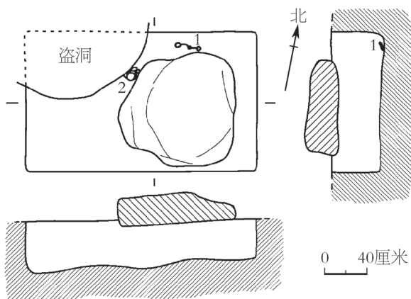
图一二 M19 平面、剖视图
