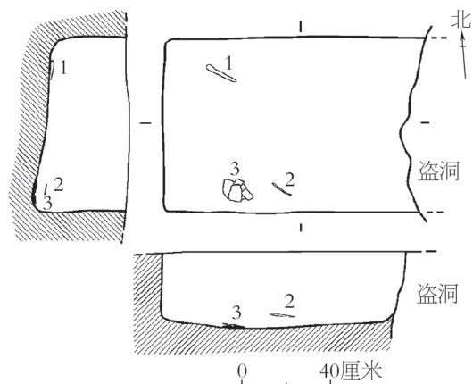
图六 M6 平面、剖视图
