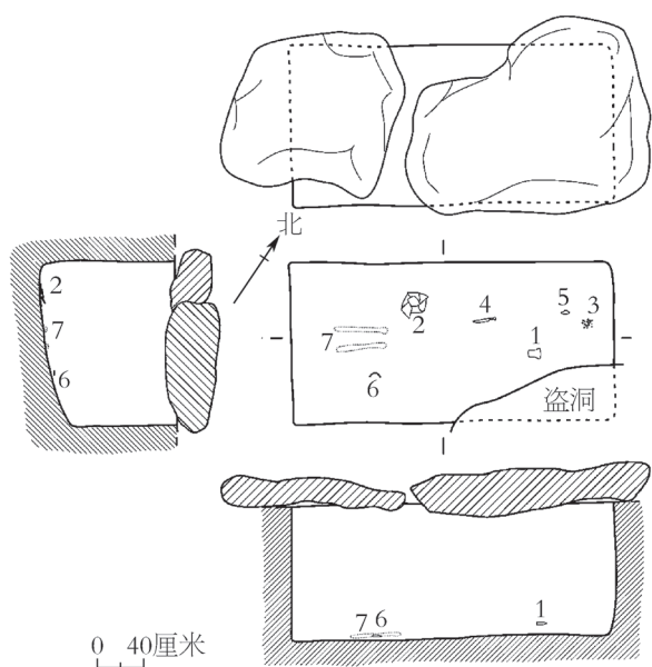
图八 M14 平面、剖视图
