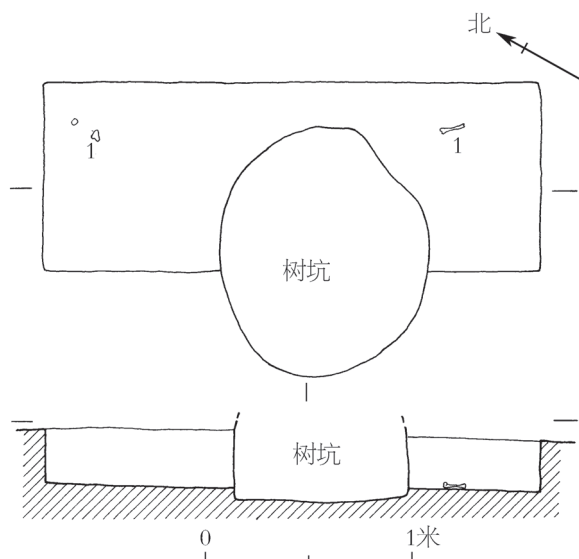
图一六 2011M35 平、剖视图
