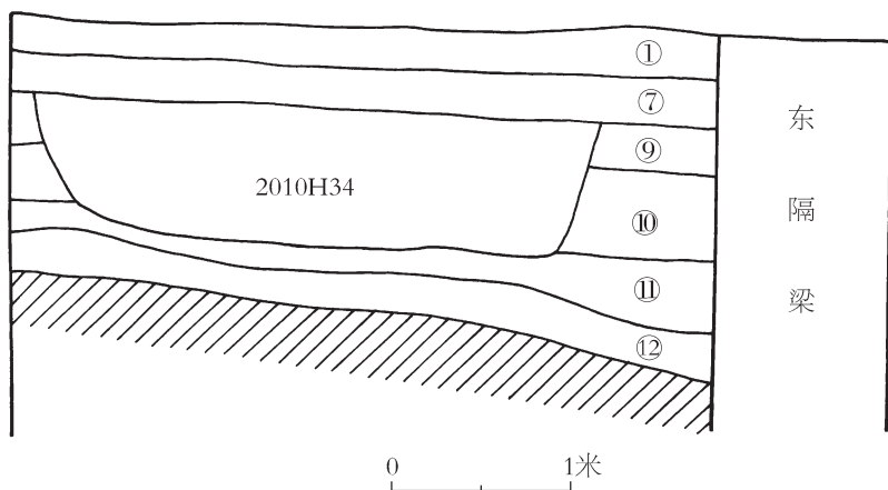
图一七 IHTS05E01 北壁剖面图
