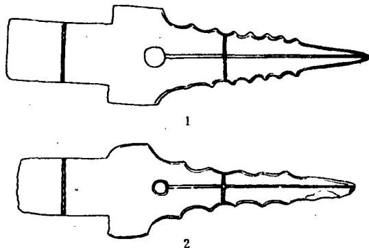
图二一 青铜戈形器(1/3) 1. B式(K2②:14附8) 2. A式(K2②:261附2)
